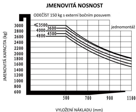
Zátěžový graf – EFL303P
