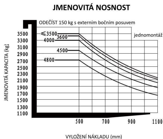
Zátěžový graf – EFL353P
