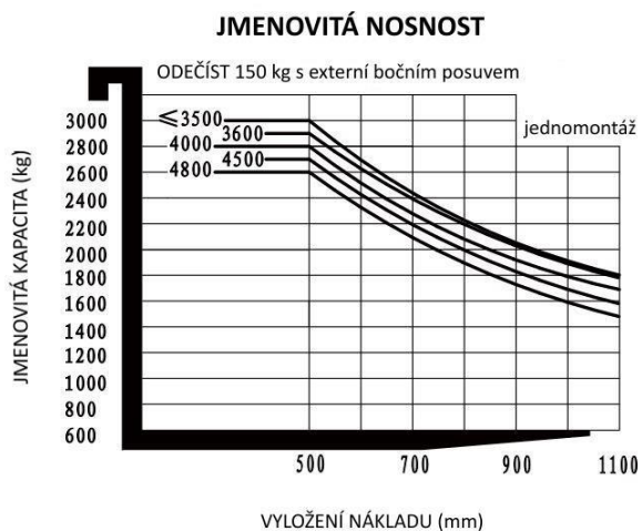
Zátěžový graf – EFL303S
