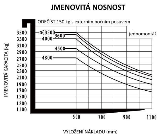
Zátěžový graf – EFL353S
