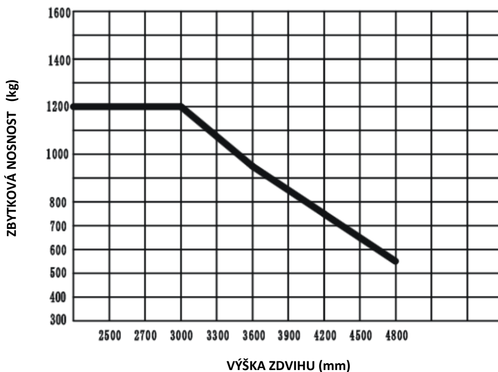
WSA121 – ZÁTĚŽOVÝ GRAF
